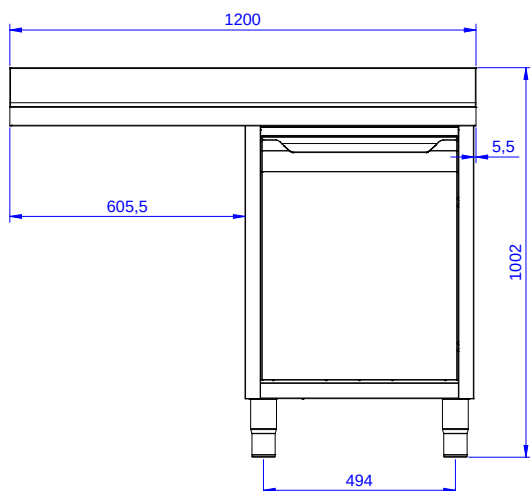
Oldalnézet
